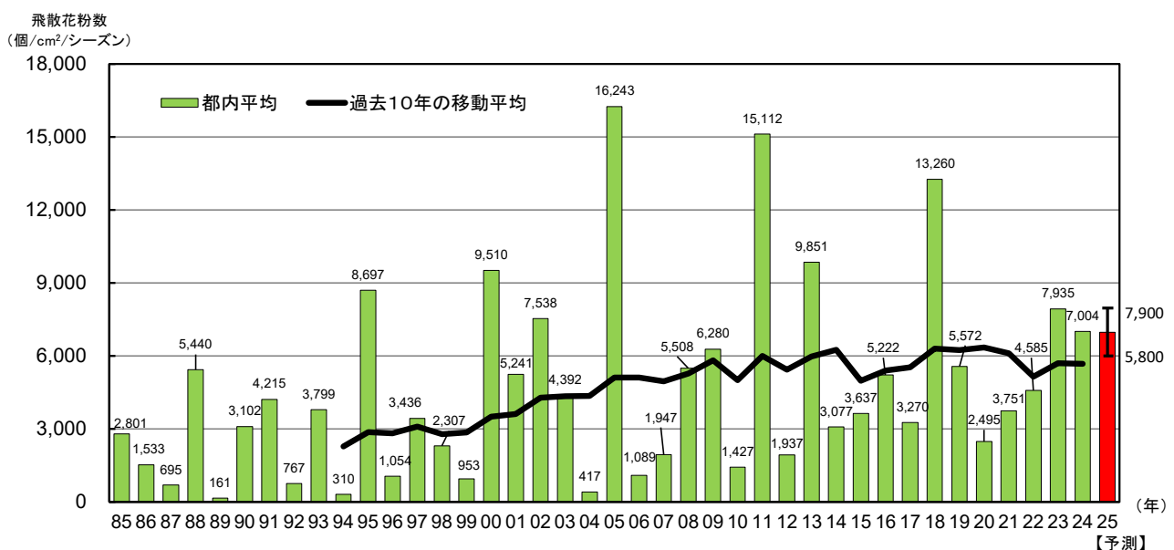
図3 飛散花粉数の経年変化※4
