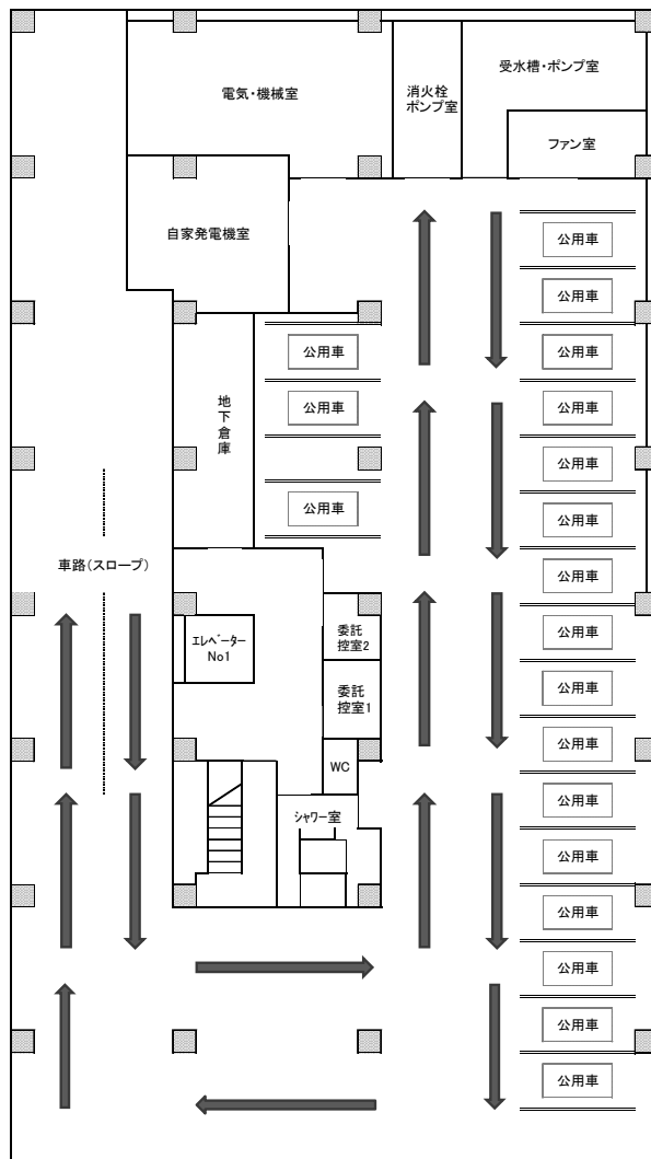
地 階
