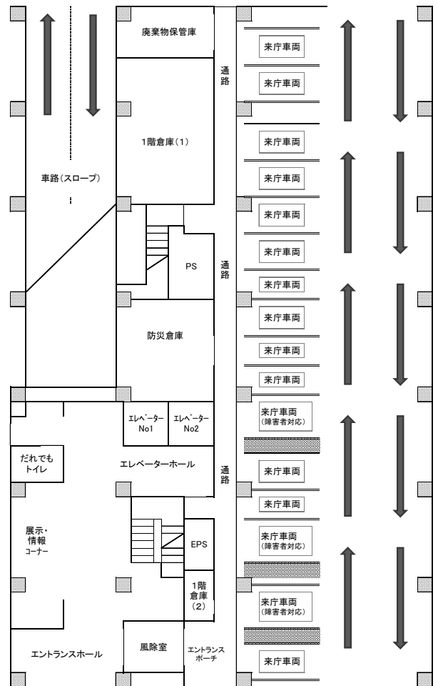
1 階
