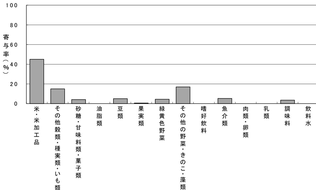
図5-1 カドミウムの一掃摂取量の寄与率(令和6年度)
