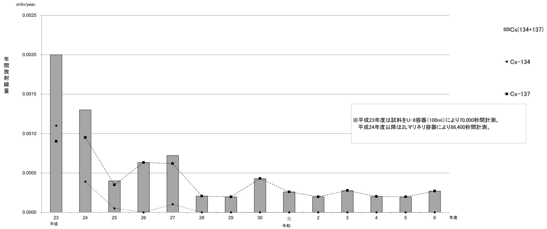
図7-2 放射性セシウムの年間放射線量の推移
