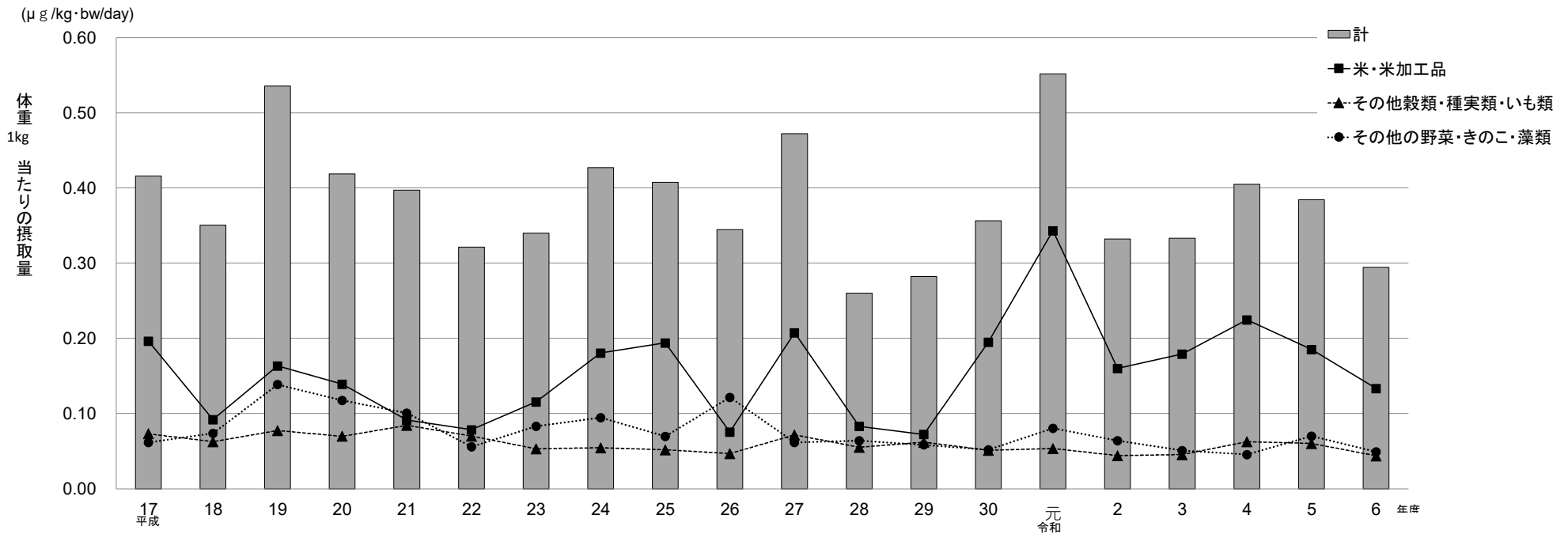
図5-2 カドミウムの一摂取量の経年変化(平成17年度～令和6年度)
