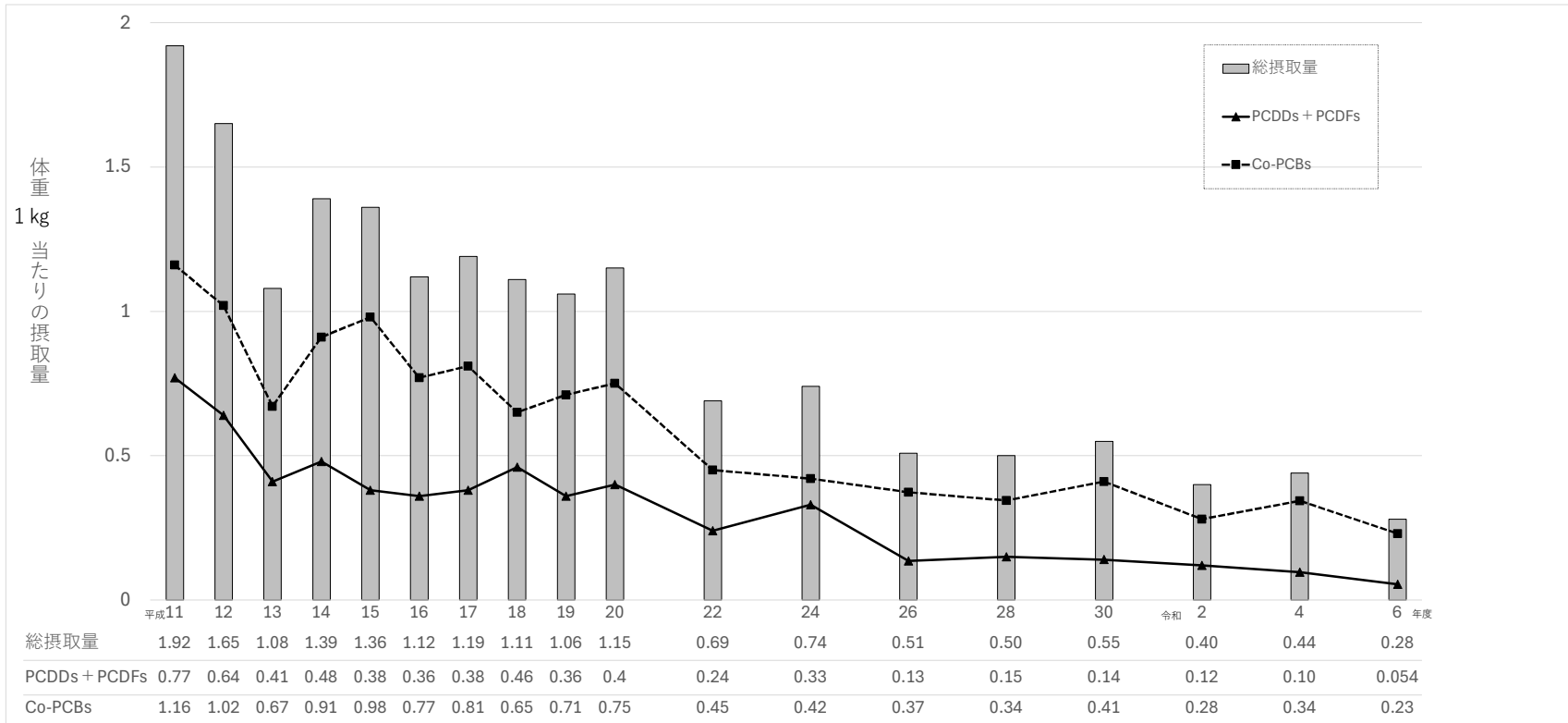
図1 ダイオキシン類の一日摂取量の推移(WHO-2006 TEF)
